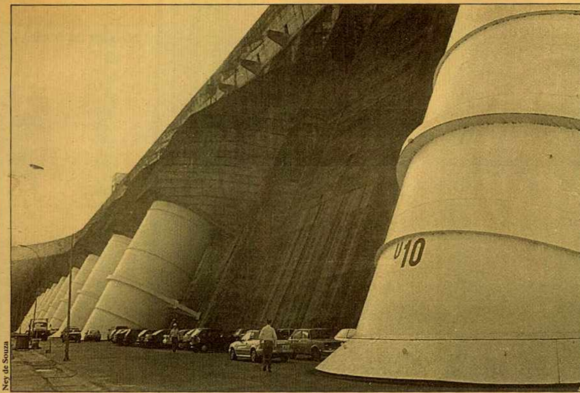
As duas novas turbinas devem estar instaladas até 2002, com capacidade total de 14 mil megawatts
