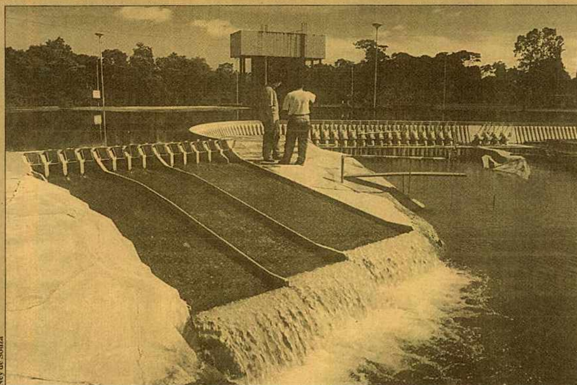
Cem vezes menor que a usina, a miniatura serviu para testes sobre a construção da hidrelétrica
