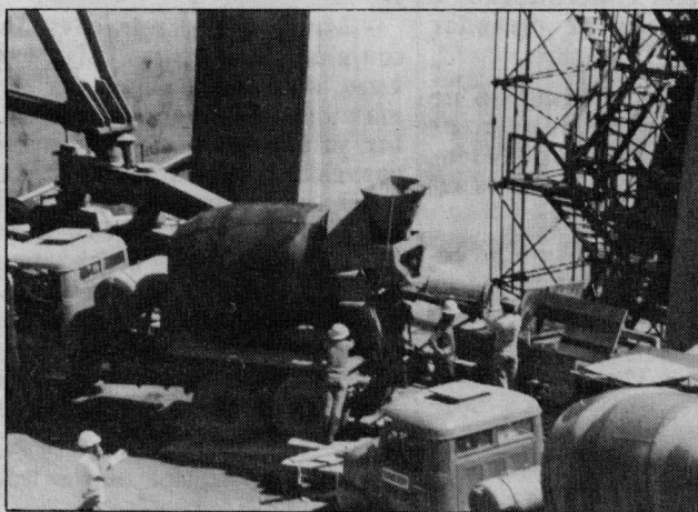
Concreto bombeável, uma alternativa encontrada para a concretagem da Casa de Força do Canal de Desvio.
