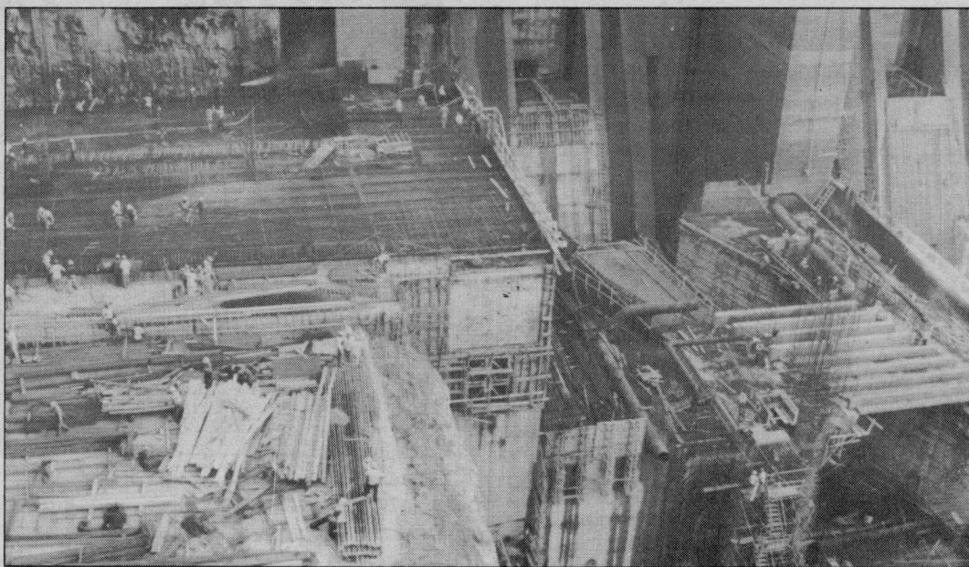
Devido a dificuldades naturais no Canal de Desvio, o recurso do concreto bombeável vem sendo bastante utilizado na Casa de Força.
