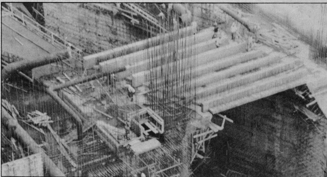
Sobre o Tubo de Sucção, as vigas premoldadas facilitam bastante os trabalhos de prosseguimento da estrutura, possibilitando ganho de tempo e economia, uma vez que se dispensa a utilização de escoramentos.
