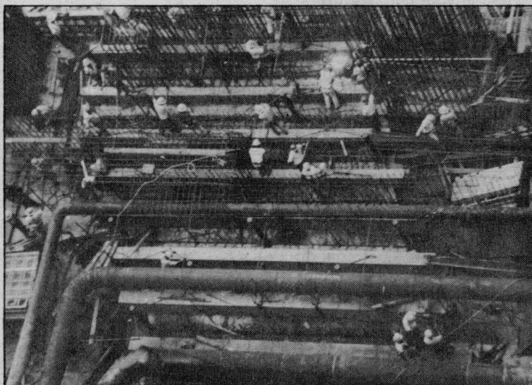
Vigas pré-moldadas foram fixadas sobre o Tubo de Sucção e Conduto Forçado da Unidade 16 e agora, facilitam o trabalho de prosseguimento da estrutura.
