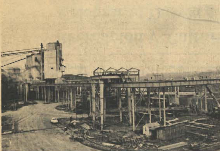
Vista geral da fase A das monovias, já em fase de conclusão.
